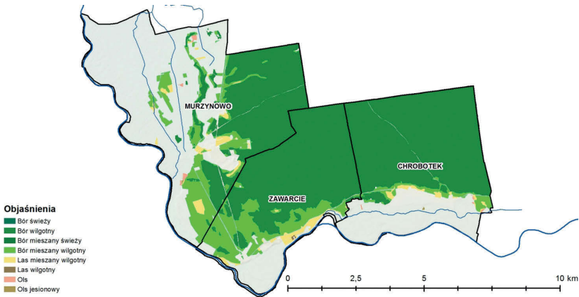
Ryc. 70. Rozmieszczenie typów siedliskowych lasu w Nadleśnictwie Skwierzyzna
