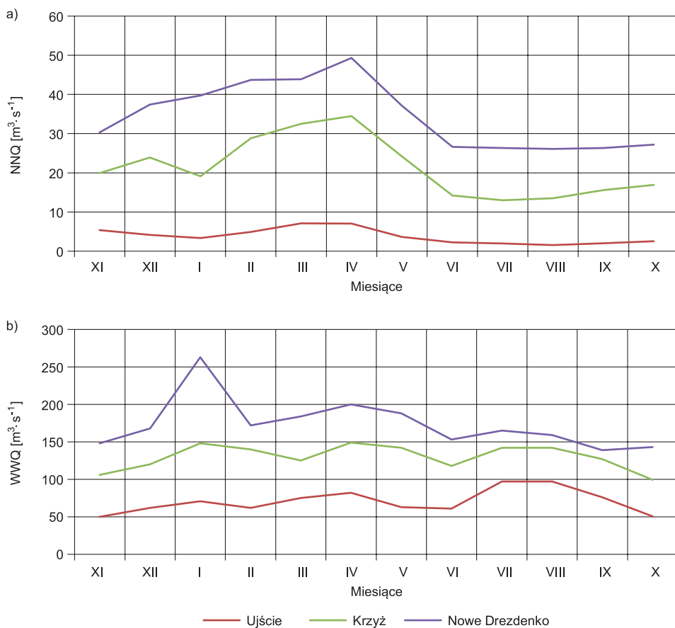
Ryc. 105. Miesięczne przepływy minimalne (a) i maksymalne (b) Noteci z wielolecia 1961–2000 na odcinku od Ujścia do Nowego Dreżdenka
