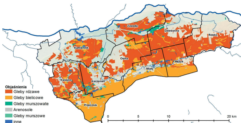
Ryc. 36. Rozmieszczenie dominujących typów gleb w Nadleśnictwie Potrzebowice
